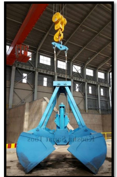
گراب کنترل از راه دور ۴,۵ متر مکعبی - ۳- دستگاه - مشتری : کارخانه مس شهر بابک
